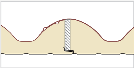
Particolare giunto tra pannelli
