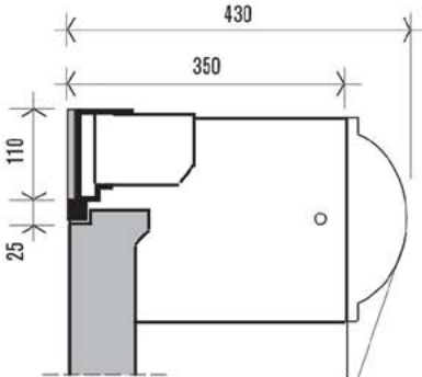
SEZIONE VERTICALE SECTION VERTICALE
