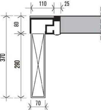
SEZIONE ORIZZONTALE SECTION HORIZONTALE
