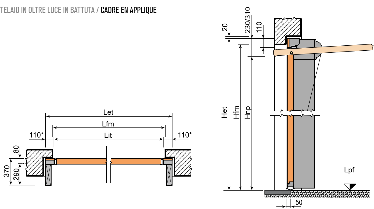
SEZIONE ORIZZONTALE SECTION HORIZONTALE
