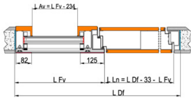
DETTAGLIO LATO SERRATURA LOCK SIDE DETAIL
