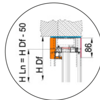
DETTAGLIO LATERALE LATERAL PANEL DETAIL
