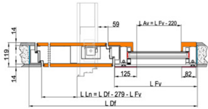
DETTAGLIO LATO CERNIERA HINGE SIDE DETAIL
