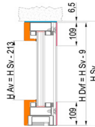
DETTAGLIO SOPRALZO TRANSOM DETAIL
