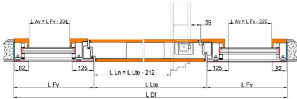
LATERALE DOPPIO DOUBLE LATERAL PANEL
