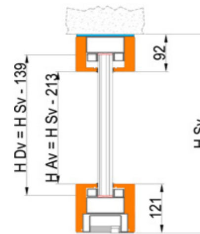
DETTAGLIO SOPRALZO TRANSOM DETAIL
