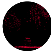
PRECISION ENHANCEMENT
