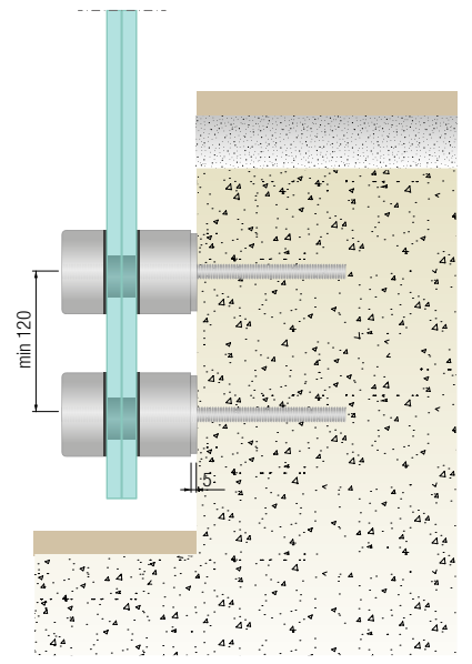
5 DAL LATO INTERNO MURETTO Fissaggio interno
