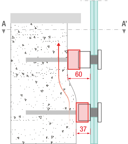
SEZIONE LATERALE (esempio di regolazione verticale)
