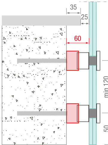
REGOLAZIONE MASSIMA Esempio con sporgenza da 35 mm
