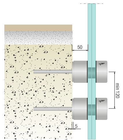
1 SENZA SPORGENZA Fissaggio esterno
