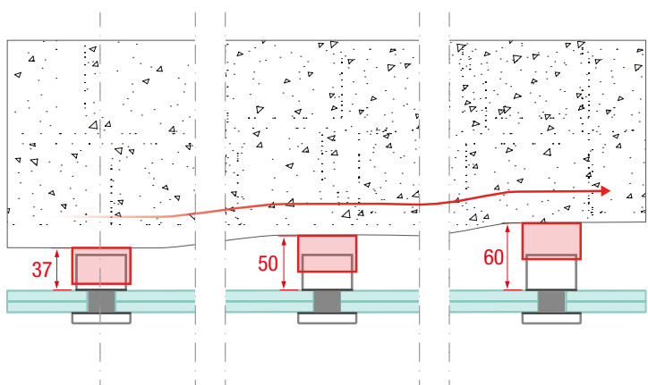
SEZIONE A-A' (esempio di regolaizione orizzontale)
