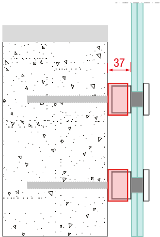
REGOLAZIONE MINIMA Esempio senza sporgenza
