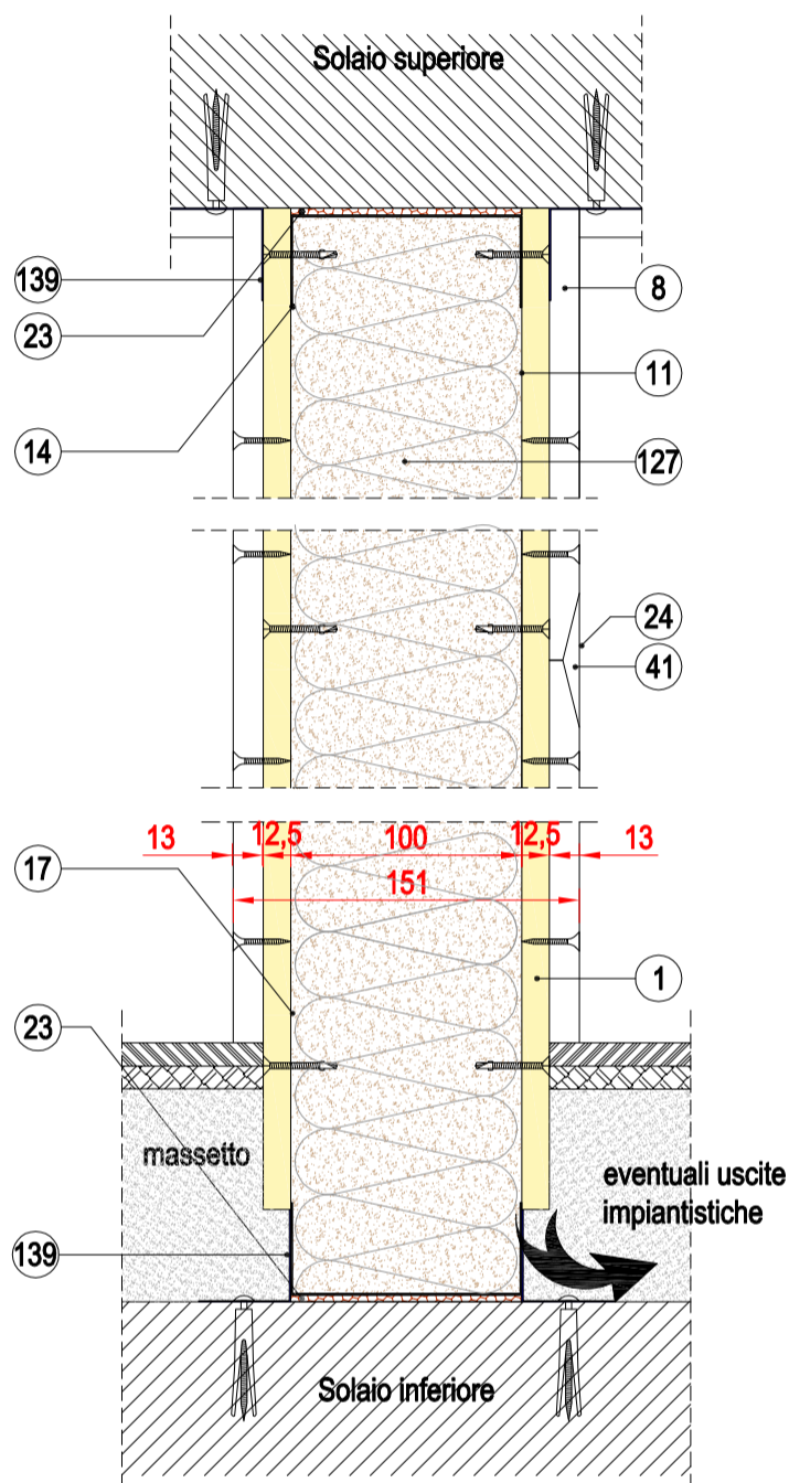
Sezione verticale
