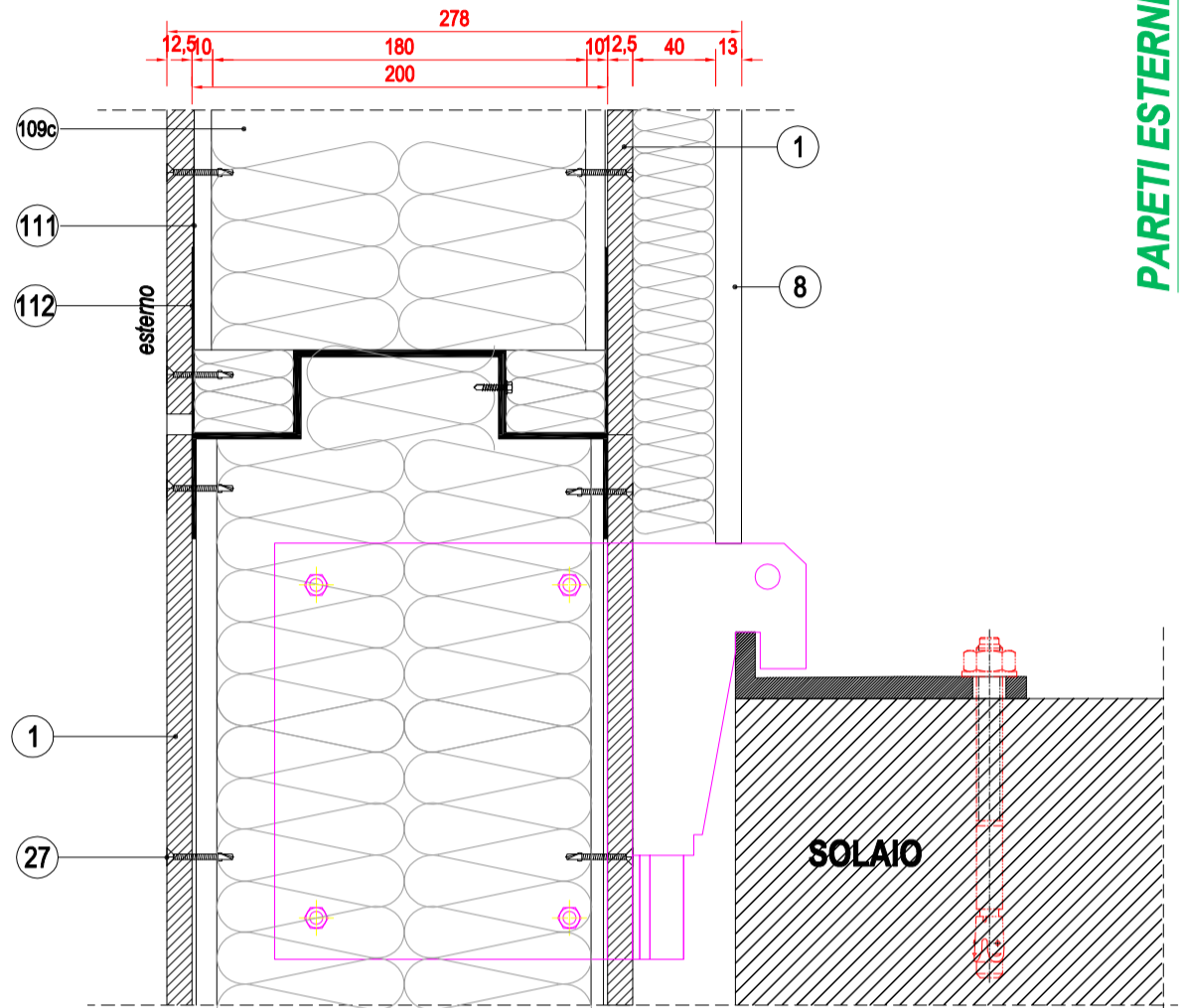
Sezione verticale su solaio
