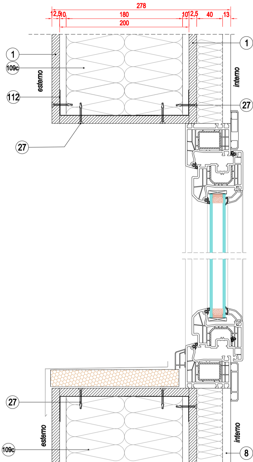
Sezione verticale su infisso
