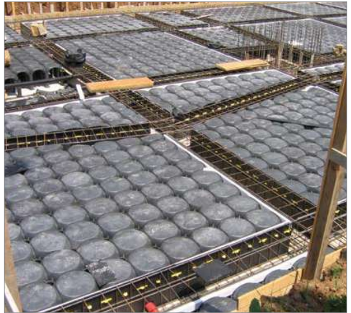
System Atlantis zusammen mit Schalung Muro
