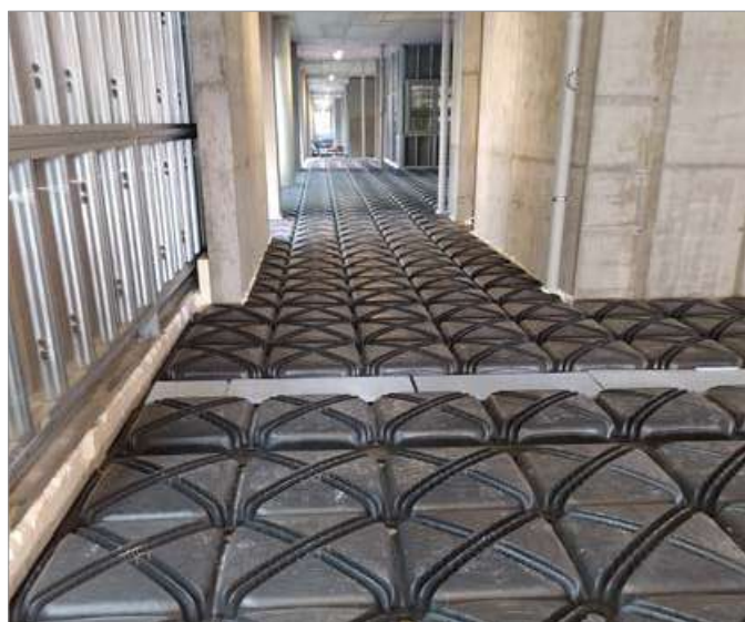
Belüftungshohlraum für Industriegebäude
