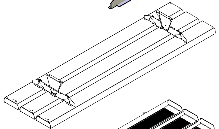
SUPPORTO DI FISSAGGIO PER N.3 TERRACE HEATER
