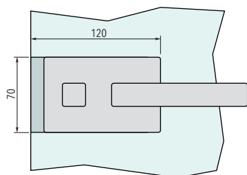
DIMENSIONI DEL BLOCCO SERRATURA
