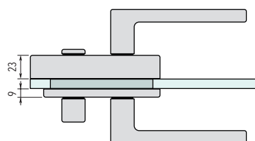
DIMENSIONI DEL BLOCCO SERRATURA
