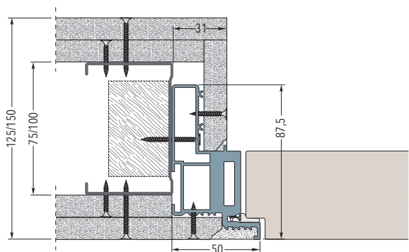
Telaio su parete in cartongesso con due lastre - Spessore parete finita 125/150 mm
