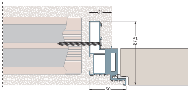
Telaio su parete per intonaco
