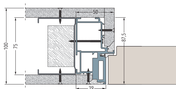
Telaio su parete in cartongesso con una lastra - Spessore parete finita 100 mm
