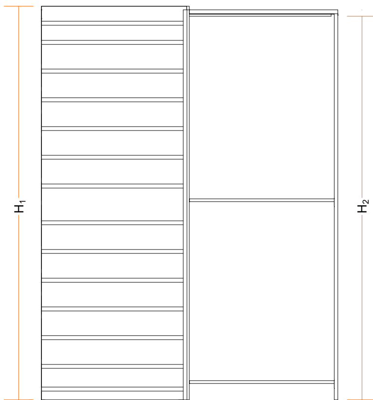
PROSPETTO
