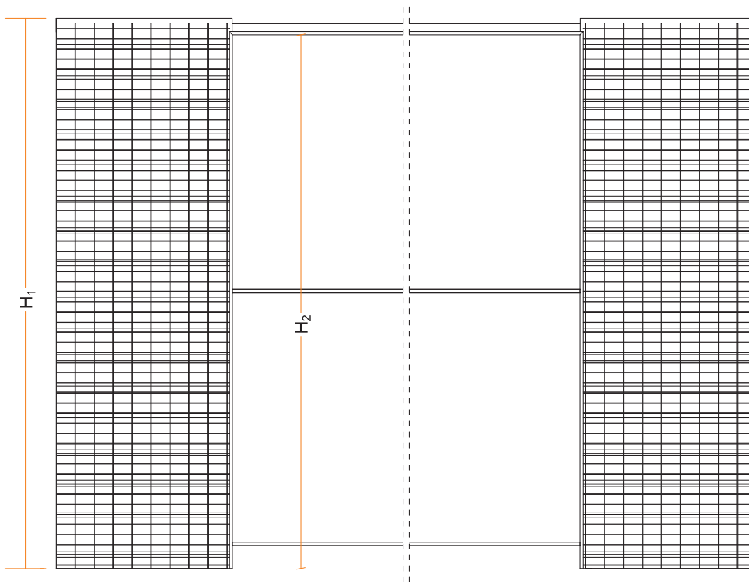
PROSPETTO
