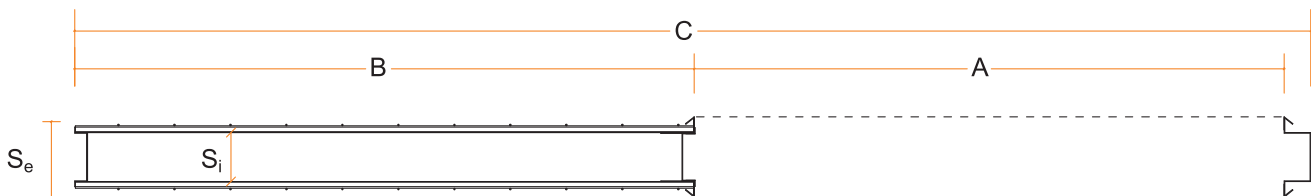
SEZIONE ORIZZONTALE
