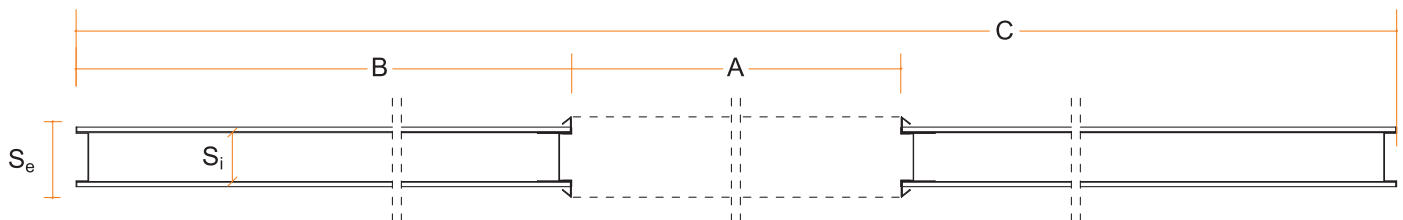
SEZIONE ORIZZONTALE
