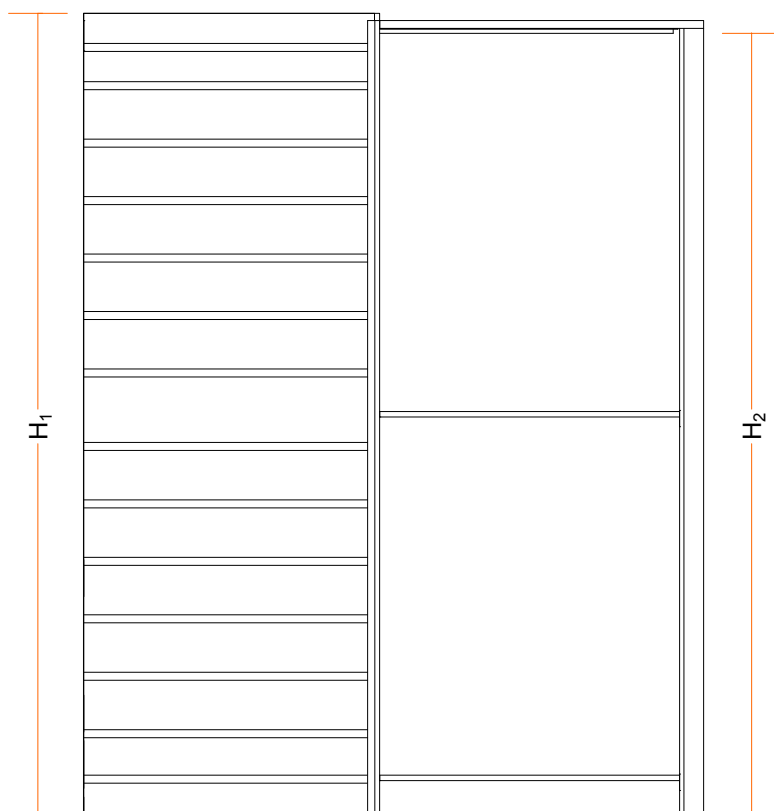
PROSPETTO
