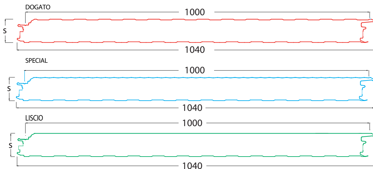
DISEGNO TECNICO Super TOP W.
