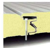
PARTICOLARE DEL GIUNTO
