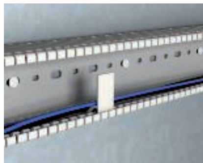
Montaggio passerella fermafilo Inserire la passerella fermafilo nella fessura laterale dei canali di cablaggio VK. Ciò facilita l'installazione del cavo e consente di fissarlo saldamente al canale VK. In tal modo la parte superiore viene posizionata senza alcuna difficoltà. In caso di eventuali installazioni successive, i cavi vengono nuovamente assicurati al canale rimuovendo la parte superiore e non ne fuoriescono.
