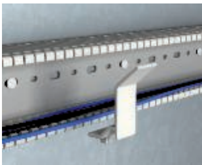
Linguette di fissaggio cavo Le linguette di tenuta dei fili possono essere adattate alla larghezza del canale. A tal scopo viene separata solo la linguetta sui punti di rottura. E' così necessaria un'unica linguetta di tenuta fili per canali di qualsiasi larghezza.
