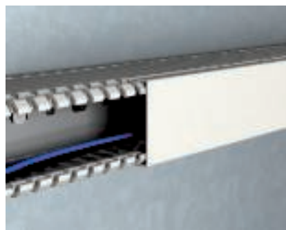
Bordo elemento superiore LKV Lo speciale bordo della parte superiore garantisce un posizionamento perfetto anche in caso di un canale di cablaggio LKV.
