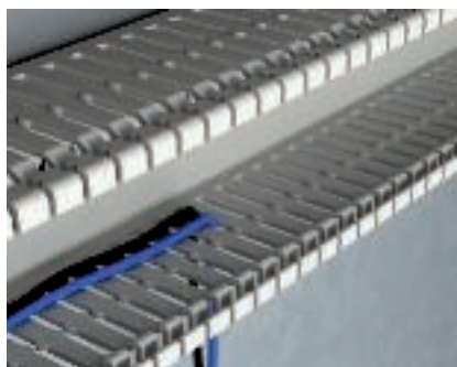
Passanti di fissaggio cavo Nelle versioni N nel ponticello laterale è inserito un passante di fissaggio che consente di bloccare il cavo nel canale di cablaggio VK.
