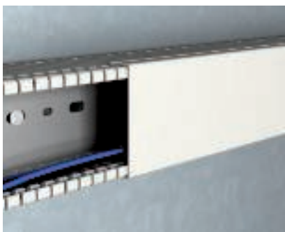
Bordo elemento superiore LK4 Una lavorazione accurata consente un'applicazione e rimozione semplificata dell'elemento superiore nonostante esso sia alloggiato saldamente.
