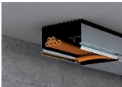
Graffe di fissaggio come supporto di montaggio per l'inserimento dei cavi con il montaggio a soffitto
