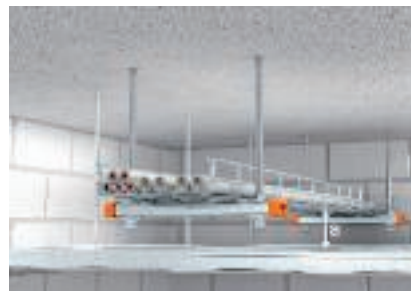
Distanza minima necessaria dal soffitto antincendio
