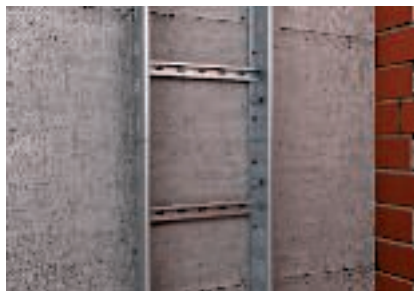
Montaggio diretto della passerella a scaletta su parete massiccia
